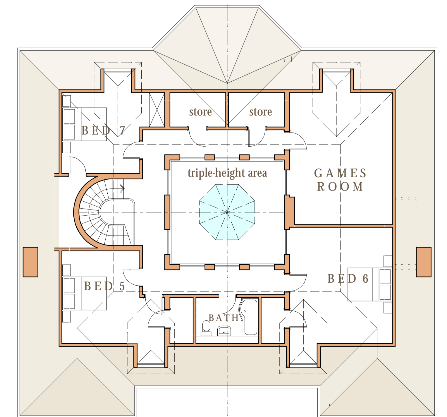
LOFT PLAN
